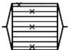
Рисунок 4 - Размещение датчиков температуры для типовых испытаний малой пористой загрузки
