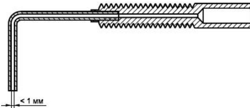
Рисунок 10 - Проходной фитинг
