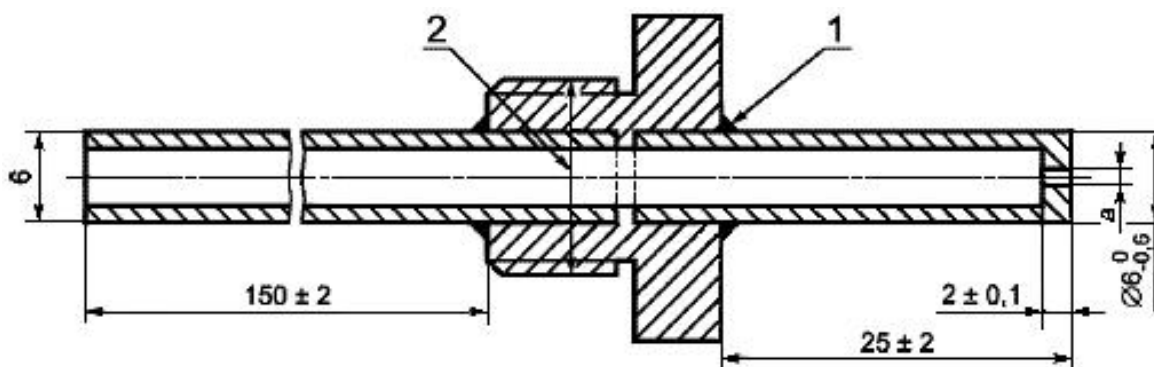
Рисунок 8 - Трубка Пито
